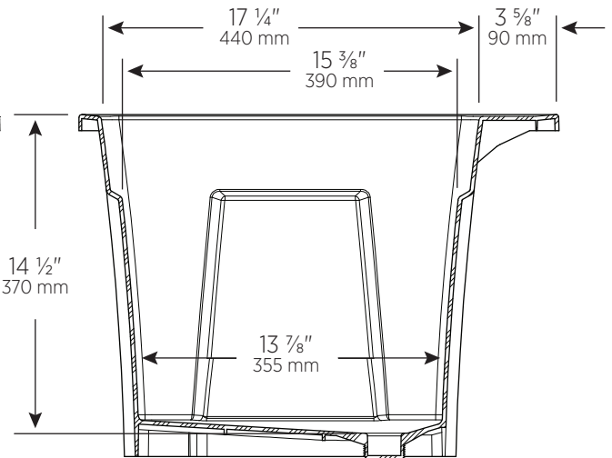
SIDE CROSS-SECTION COUPE TRANSVERSALE DE COTÉ
