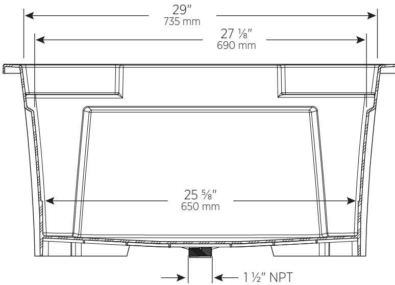
FRONT CROSS-SECTION COUPE TRANSVERSALE DE FACE
