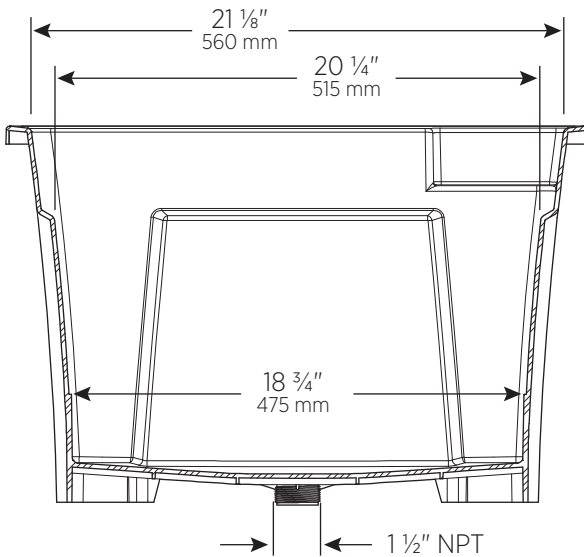
FRONT CROSS-SECTION COUPE TRANSVERSALE DE FACE
