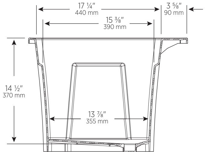
SIDE CROSS-SECTION COUPE TRANSVERSALE DE COTÉ
