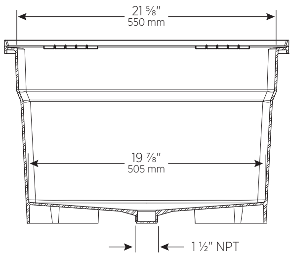
FRONT CROSS-SECTION COUPE TRANSVERSALE DE FACE
